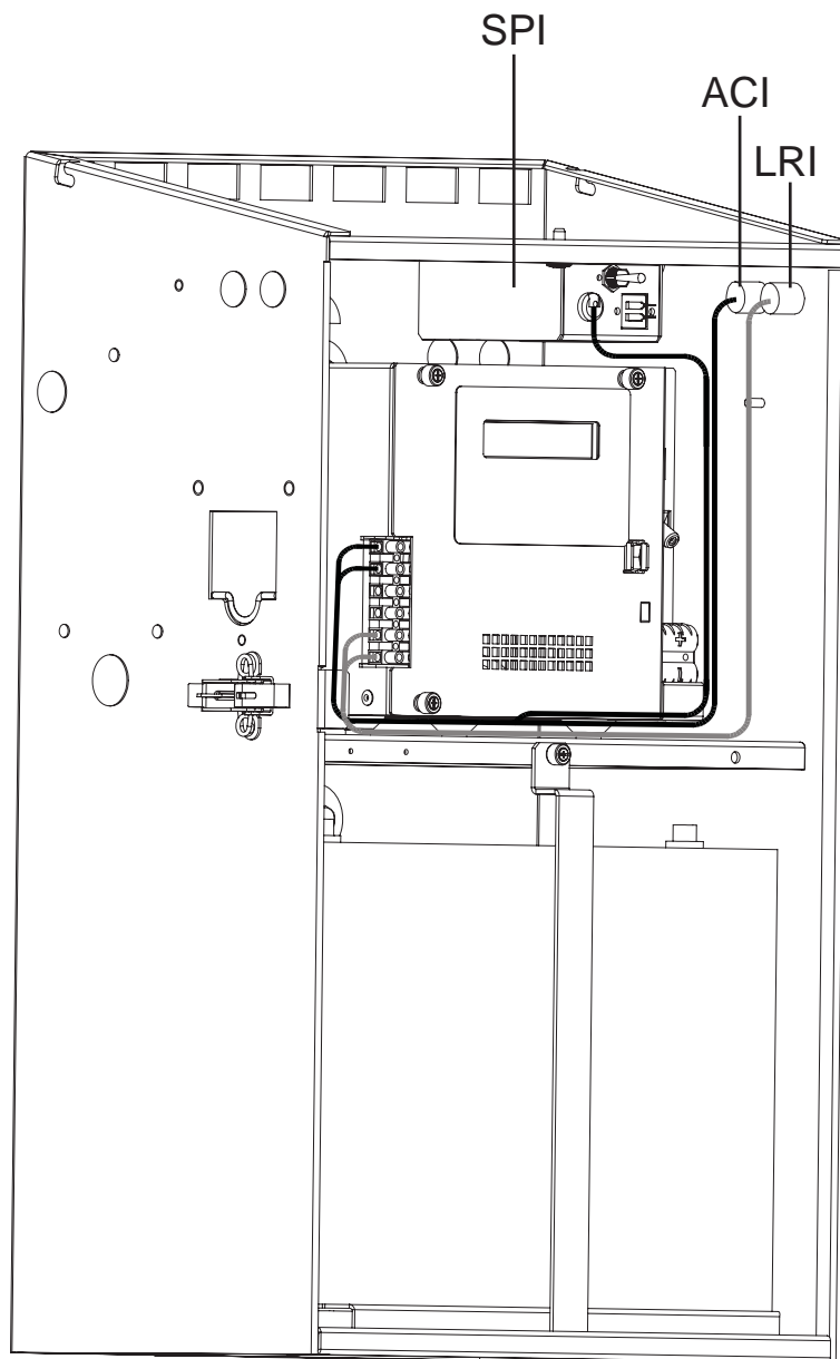
Fig. 2-3, Conexión ACI/LRI
