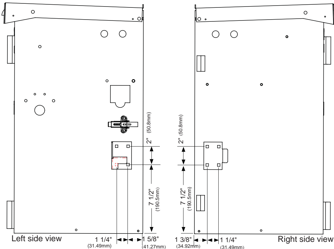
Fig. 1, PWE-3 Enclosure
